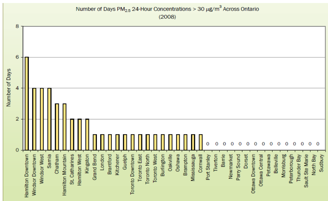
Gráfica 5.2.6. Número de días en los que las concentraciones de PM 2.5 en 24 hrs. son mayores de 30 µg/m³ en centros de población de Ontario, en 2008
